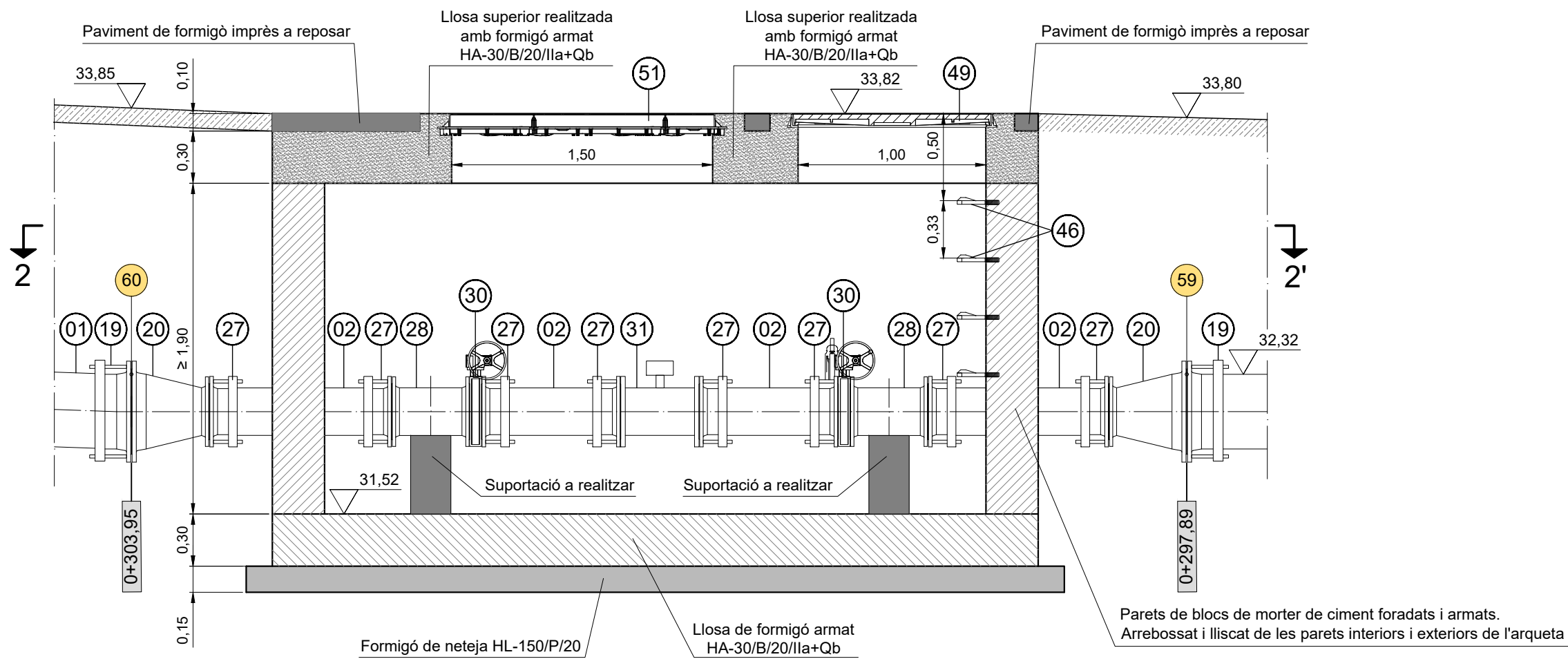
ARQUETA A-3 Secció 1-1'
