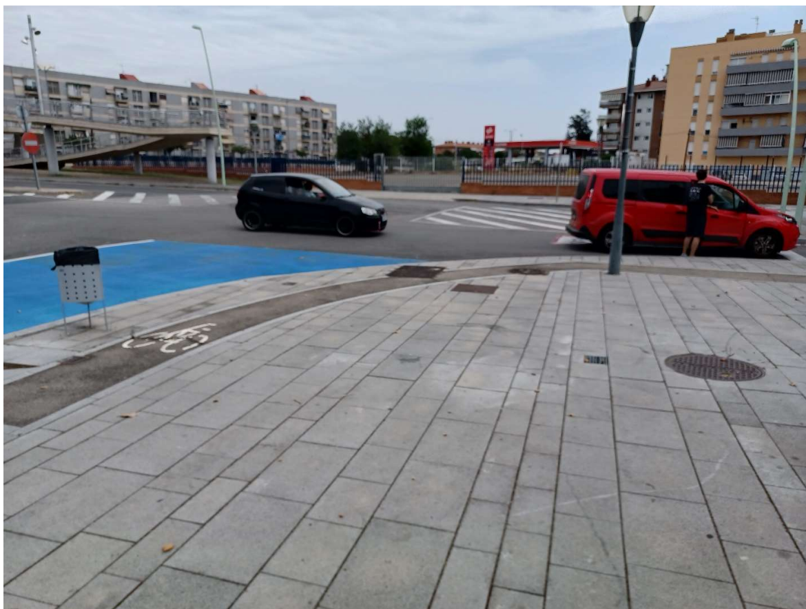
FOTO Nº 12: Vista del punt on finalitzarà un dels dos punts de connexió, del punt on es connectarà la canonada d'aigua existent de fosa dúctil de 200 mm de diàmetre a la nova canonada també de fosa dúctil de 400 mm de diàmetre.
