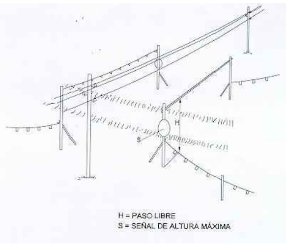
PÒRTIC DE BALISAMENT DE LÍNIES ELÈCTRIQUES AÈRIES
