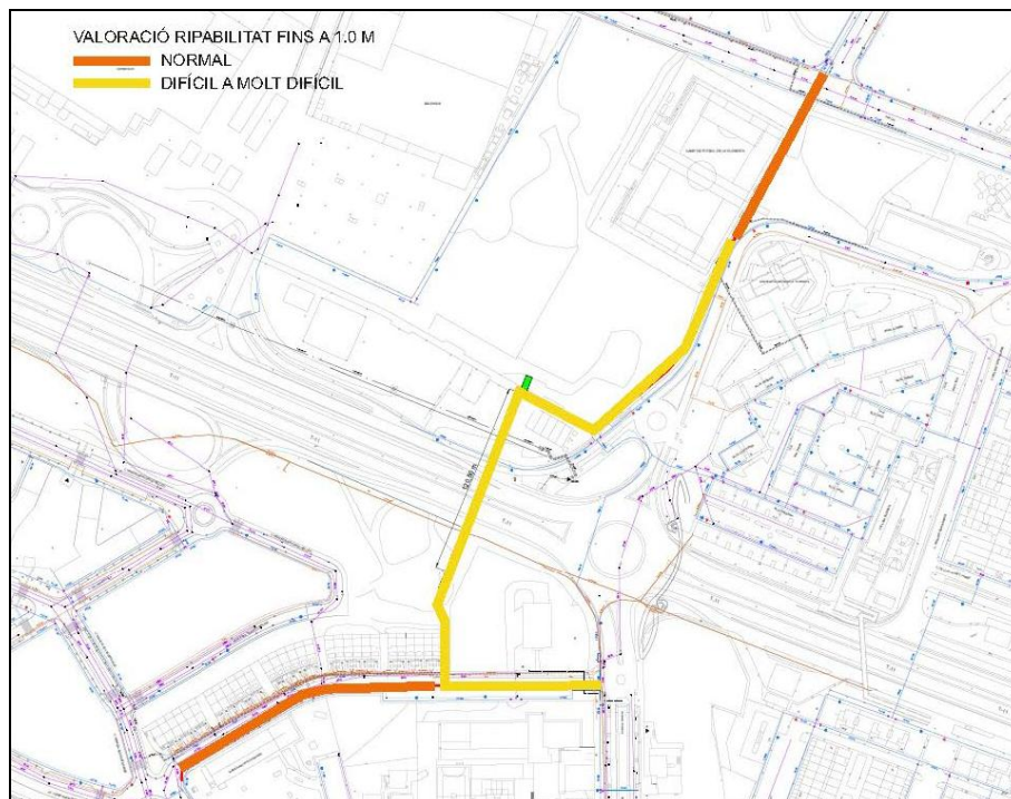
Imatge 8-2.- Valoració de la ripabilitat de 0.0 a 1.0 m
