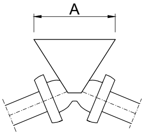
COLZE DE 45° PLANTA
