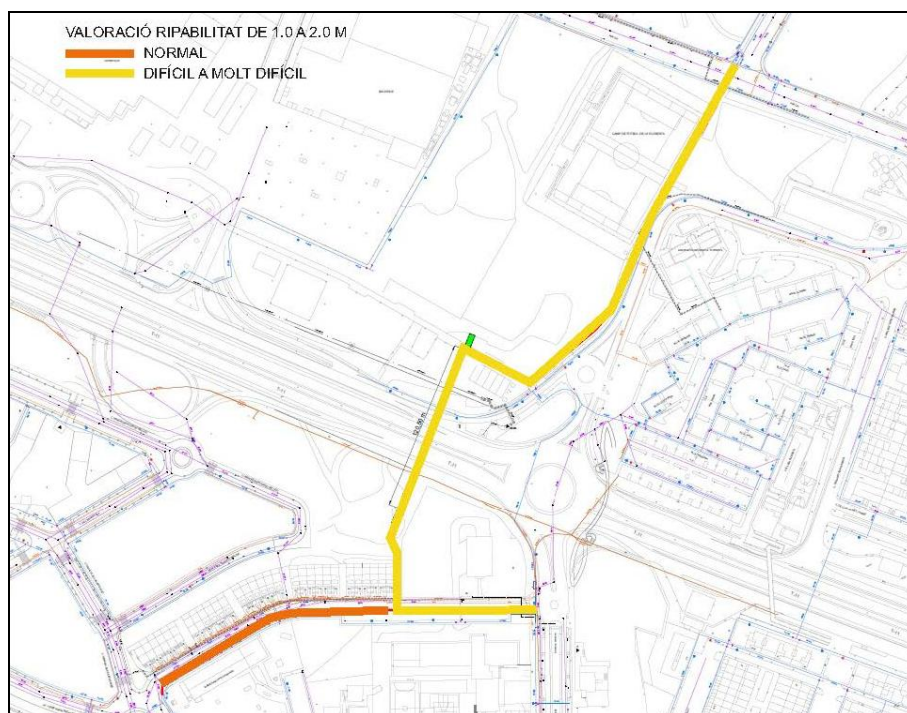
Imatge 8-3.- Valoració de la ripabilitat de 1.0 a 2.0 m
