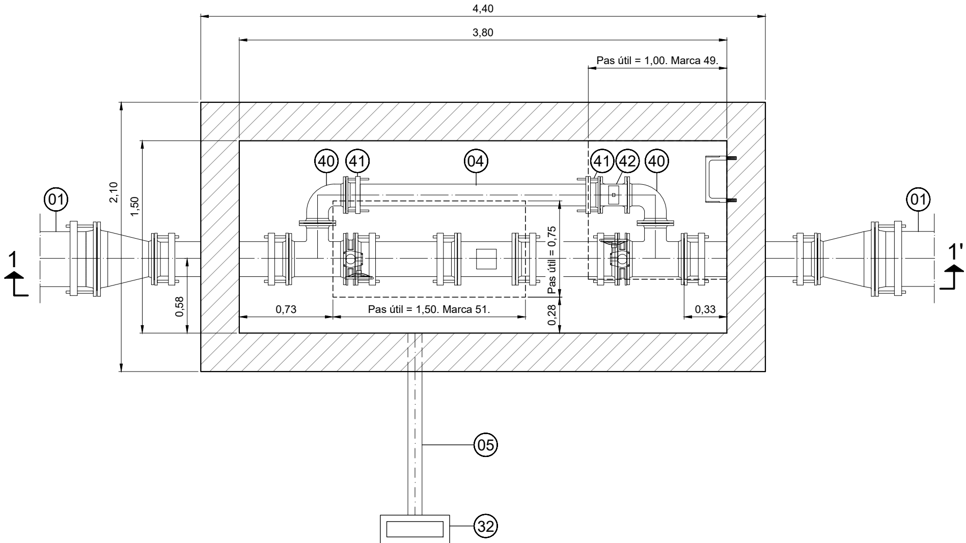
ARQUETA A-3 Secció 2-2'
