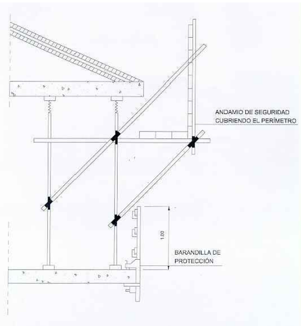
PLATAFORMA AL CANTELL DE LA COBERTA
