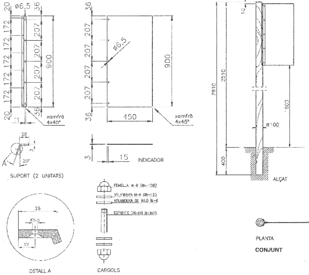
SENYAL AMB BANDEROLA 450x900mm
