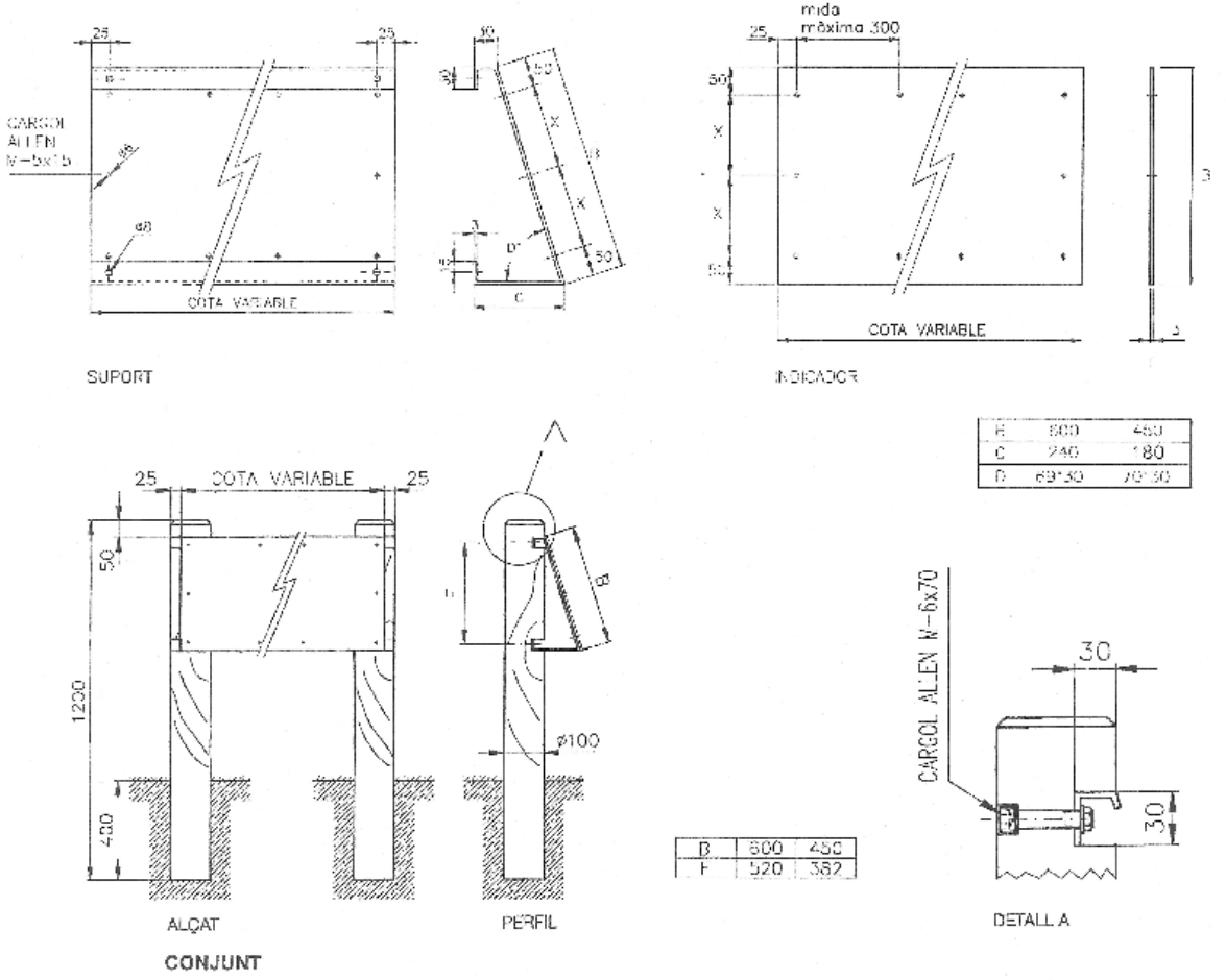
SENYAL AMB DOBLE SUPORT BAIX 900x600mm
