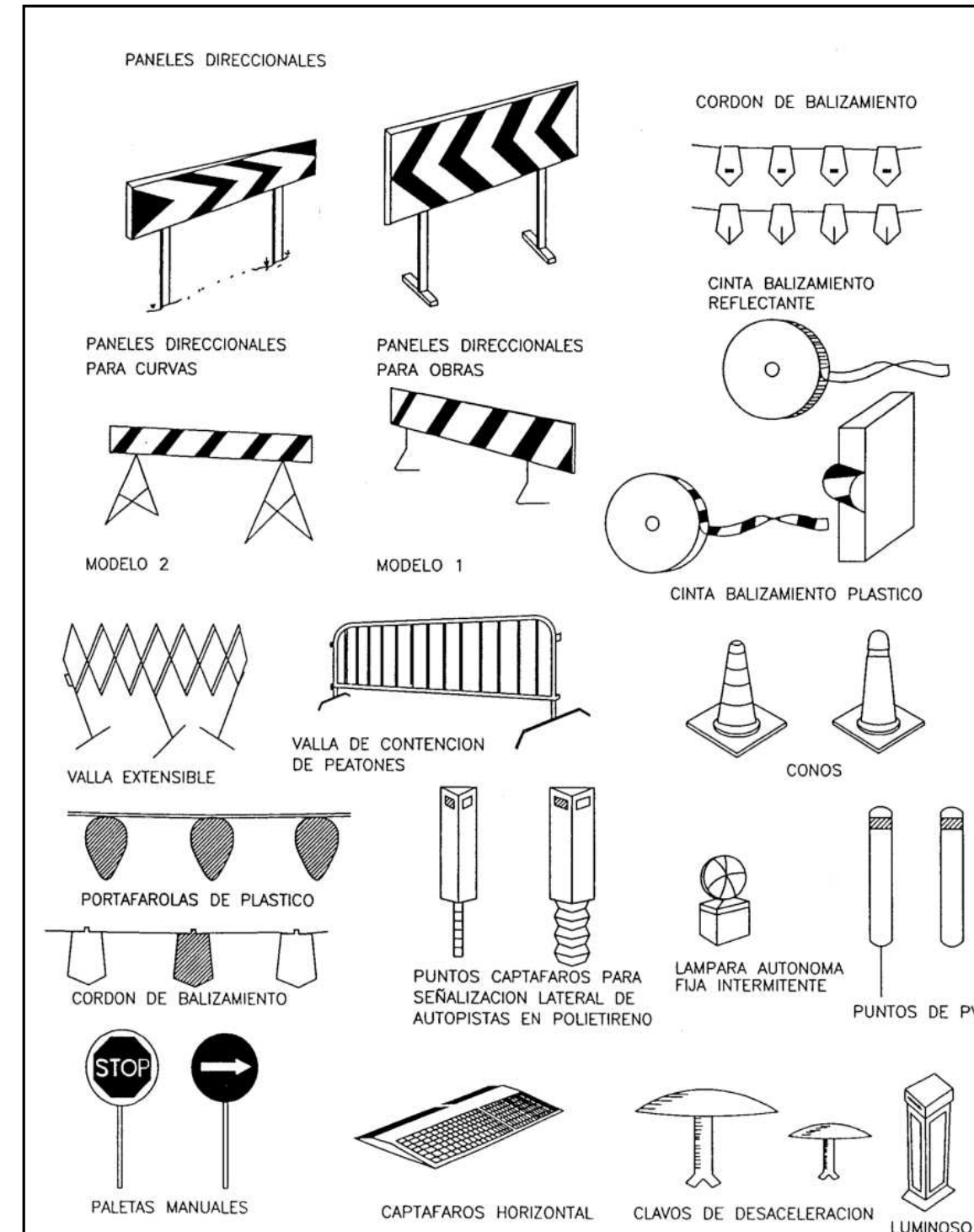
Figura 6. Elementos auxiliares de senyalització
