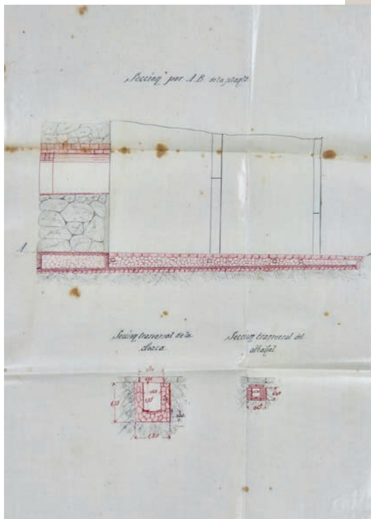
Projecte de l'arquitecte Ramon Salas per fer una obertura a la muralla per eliminar aigües brutes i una finestra de ventilació, posteriorment es va obrir la porta que van obligar a tapiar. 1883. (AHCT, expedient 2/84).
