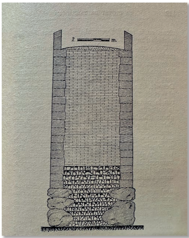
Reconstrucció de la secció de la muralla amb base megalítica, reble de pedres i terra. Part superior de carreus amb reble de toves. A: La muralla de Tarragona, Joan Serra Vilaró. 1949 (BHMT).
