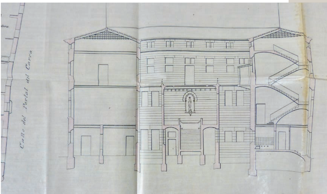
Projecte del col·legi Lestonnac, arquitecte Francisco Borràs, 1890. (AHCT)
