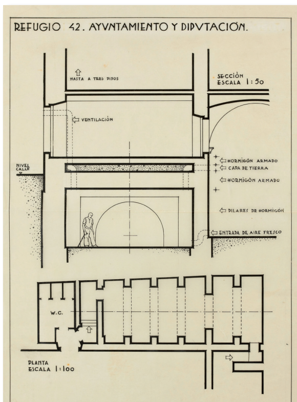
Plànol del refugi 42 interior de l'Ajuntament. AHCT/L'Arxiu
