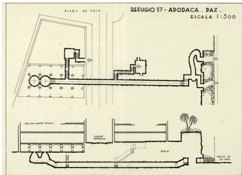
Plànol del refugi 57. AHCT
